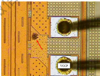
芯片内部静电损伤
