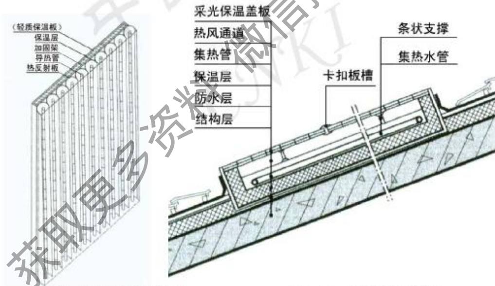
图5-48 太阳能保温墙板 [149]
