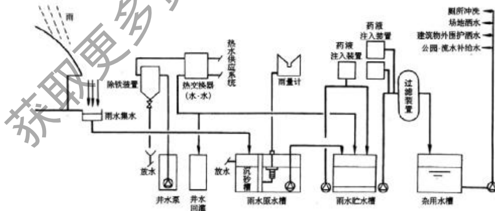
图5-80 出云穹顶雨水和井水利用系统 [22]
