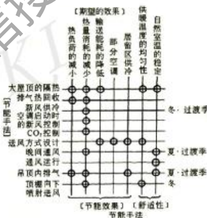
图1-8 东京体育馆节能对策 [22]
