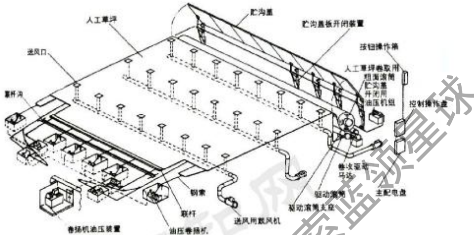
图5-87 大阪穹顶大型草坪卷取装置 [107]
