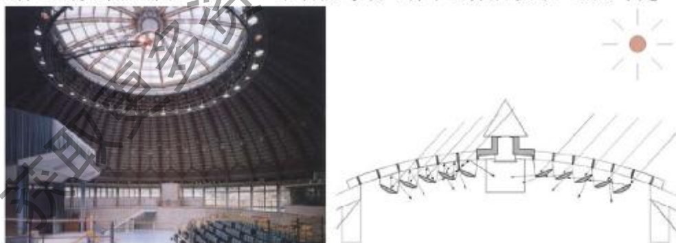
图5-68 一户町穹顶内遮阳分析
