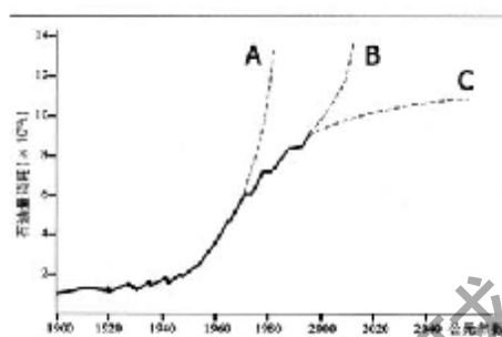
图1-3 世界能源消耗曲线图
