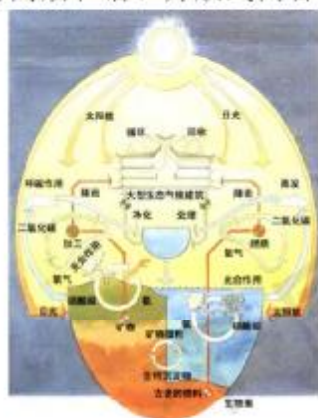
图1-1 生态系统循环示意图 [7]
