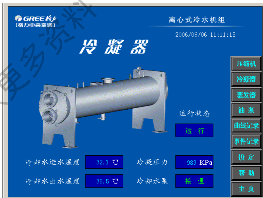
冷凝器界面
