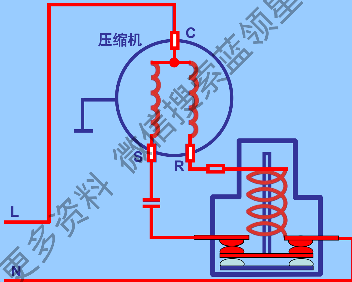
重锤式启动继电器接线示意图：
