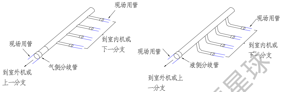
分歧集管示意圖
