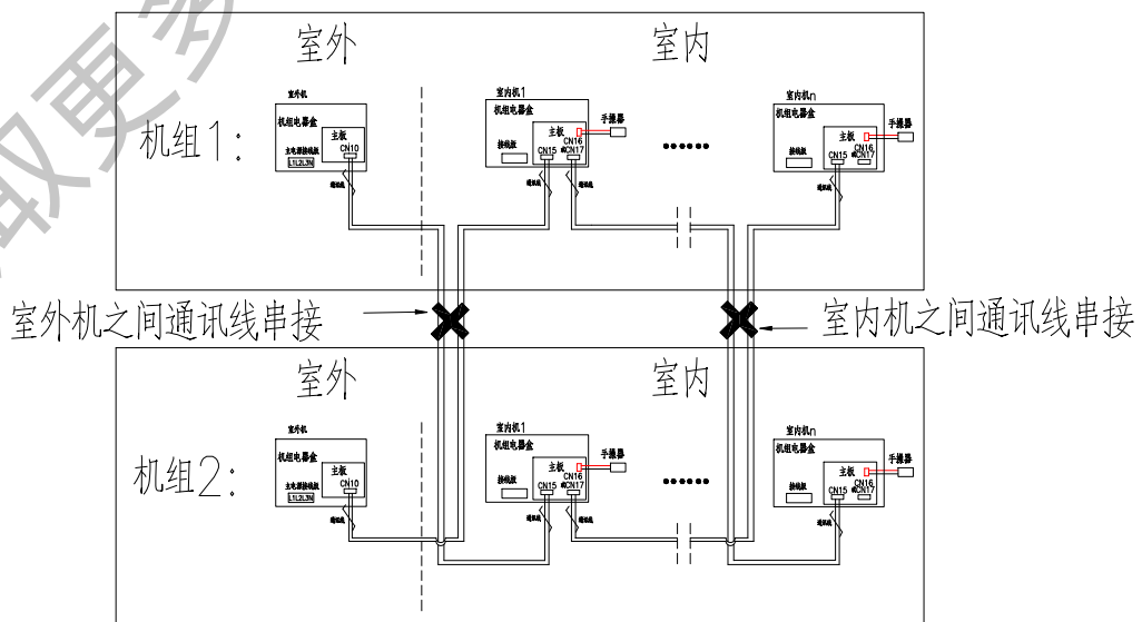
多套多联机组时通讯线的连接（正确）
