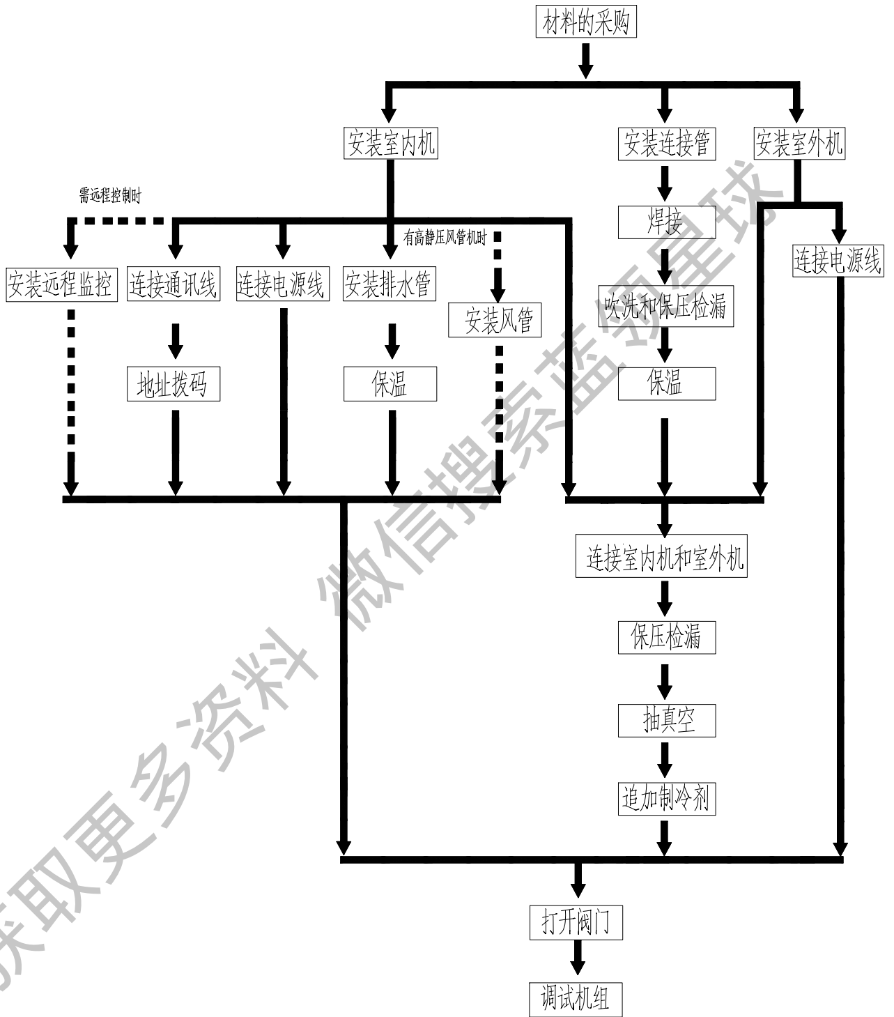
安装流程图：
