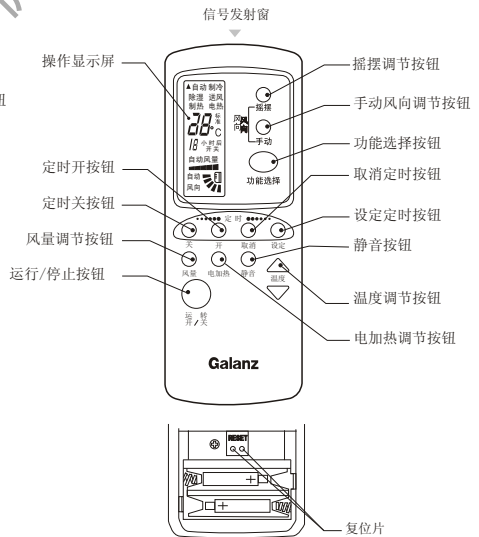
冷暖电辅助加热型遥控器
