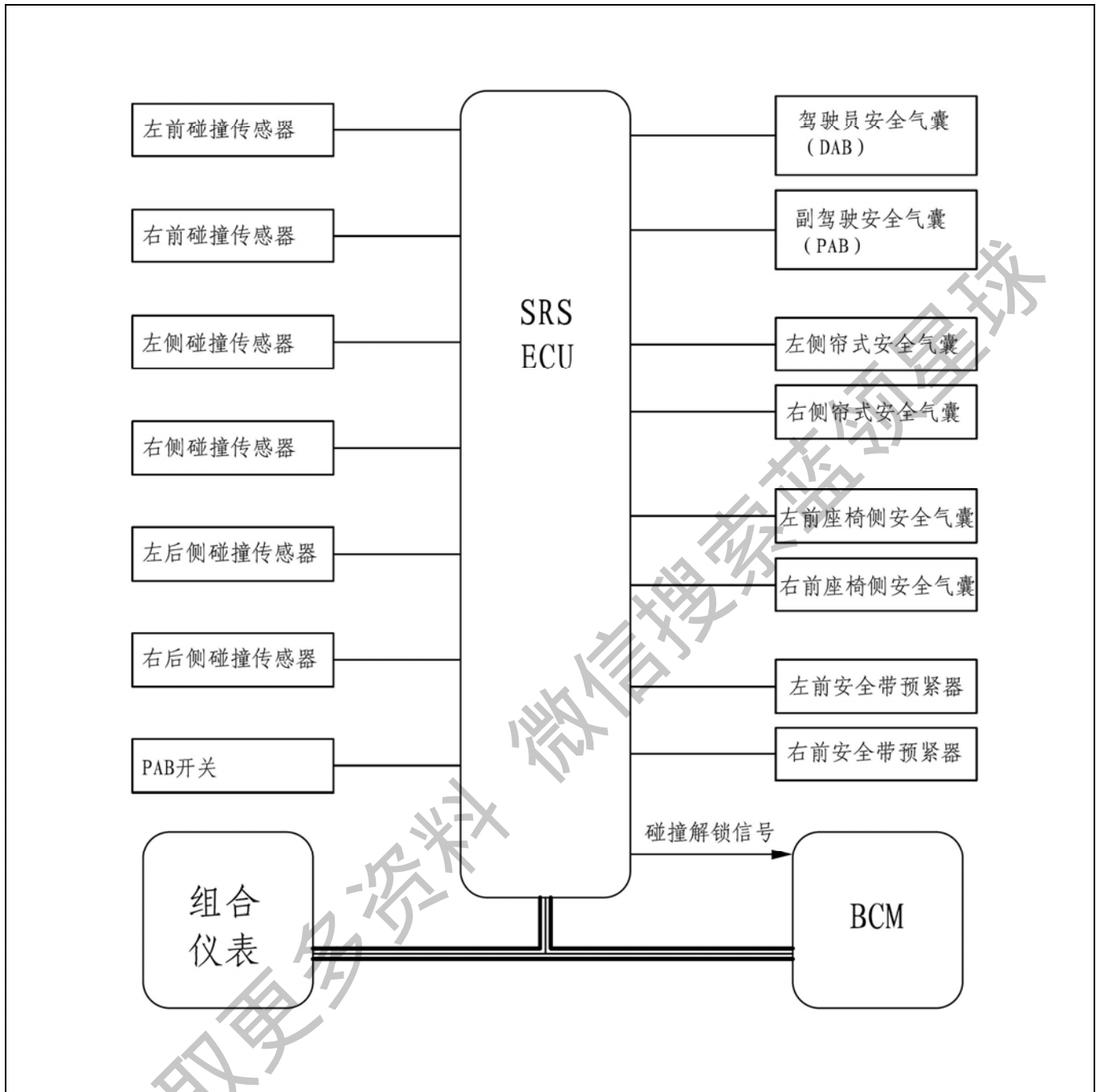
系统框图
