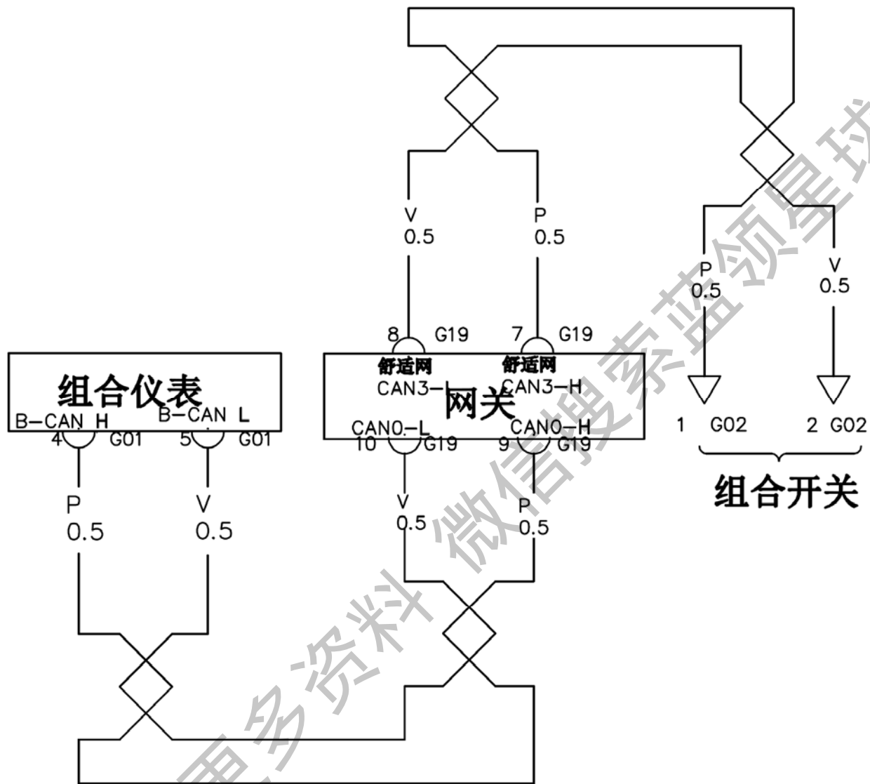
电路图
