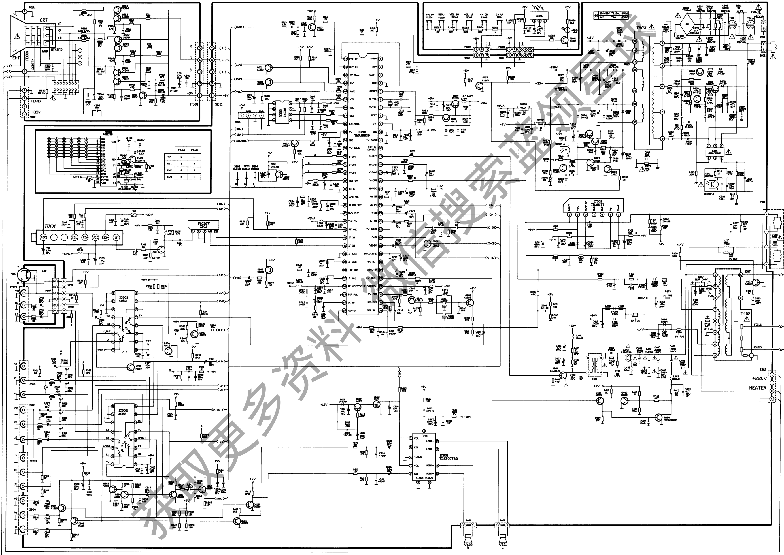
29A1 型彩色电视机电路原理图
