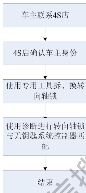
图3 更换转向轴锁流程图
