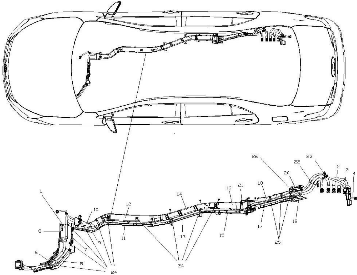
图 8.11 高压电缆总成
