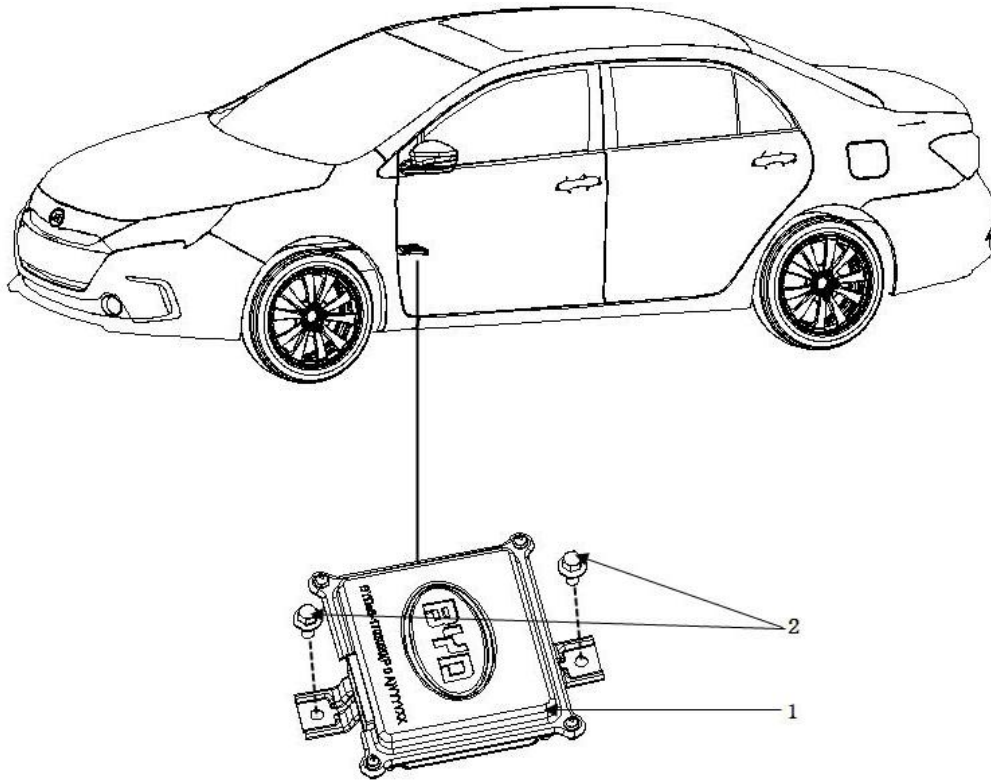
图 8.14 档位控制器
