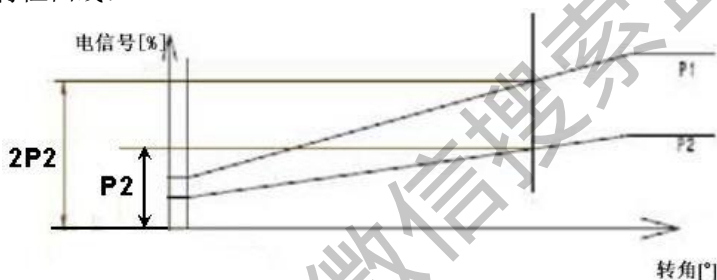
图3-37传感器电信号特性曲线
