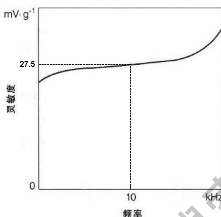
图3-29 特性曲线图
