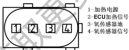
图3-12 上游氧传感器电气原理图
