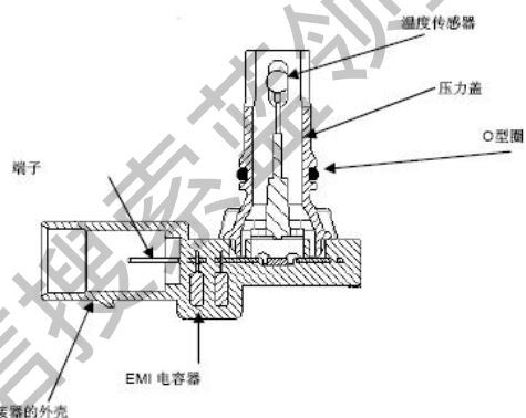
图3-4 进气压力温度传感器剖面图
