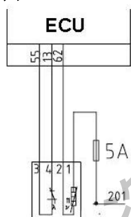
图3-12 上游氧传感器电气原理图
