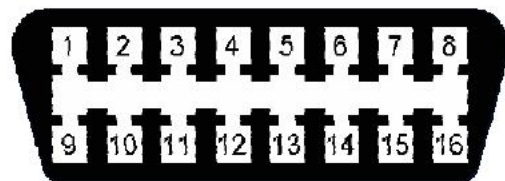
图2.5 ISO9141-2 标准诊断接头 ECU 通过“CAN”线可与外接诊断仪进行通信，并可进行如下操作：
