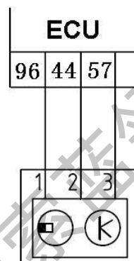
图3-23 相位传感器电气原理图
