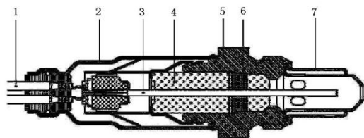
1导线 2保护套 3平面传感元 4导线 5传感器座 6密封圈 7双层保护管 图3-14 氧传感器结构图
