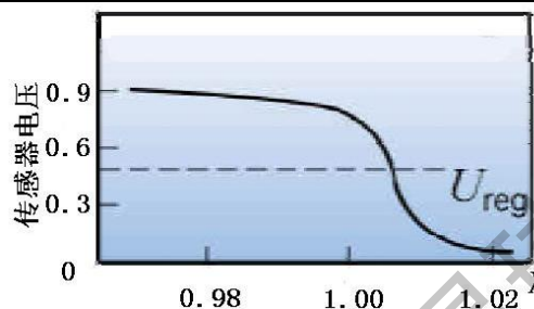
\lambda < 1 : 混合气浓 (氧不足) \lambda > 1 : 混合气稀 (氧过量)
