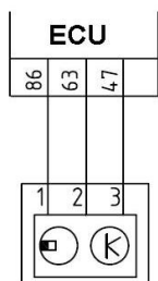
图3-19 曲轴位置传感器电气原理图
