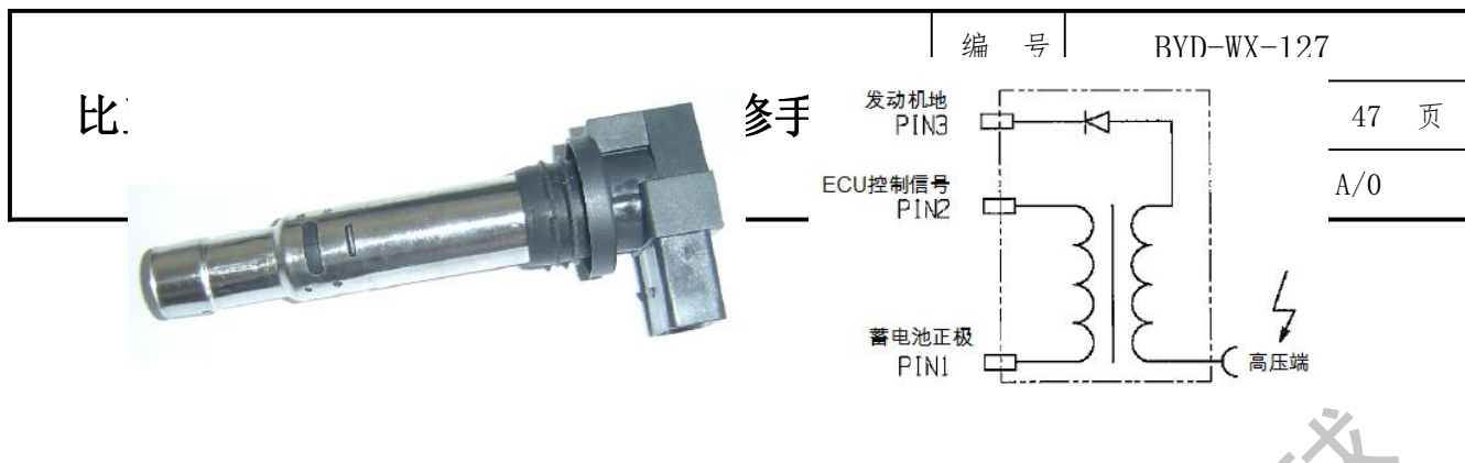
图3-57 单火花点火线圈
