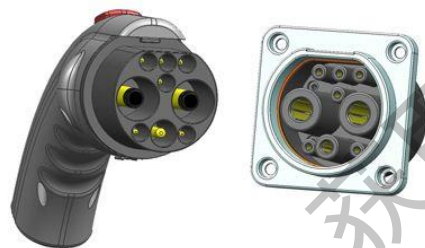
国际标准慢充接口
