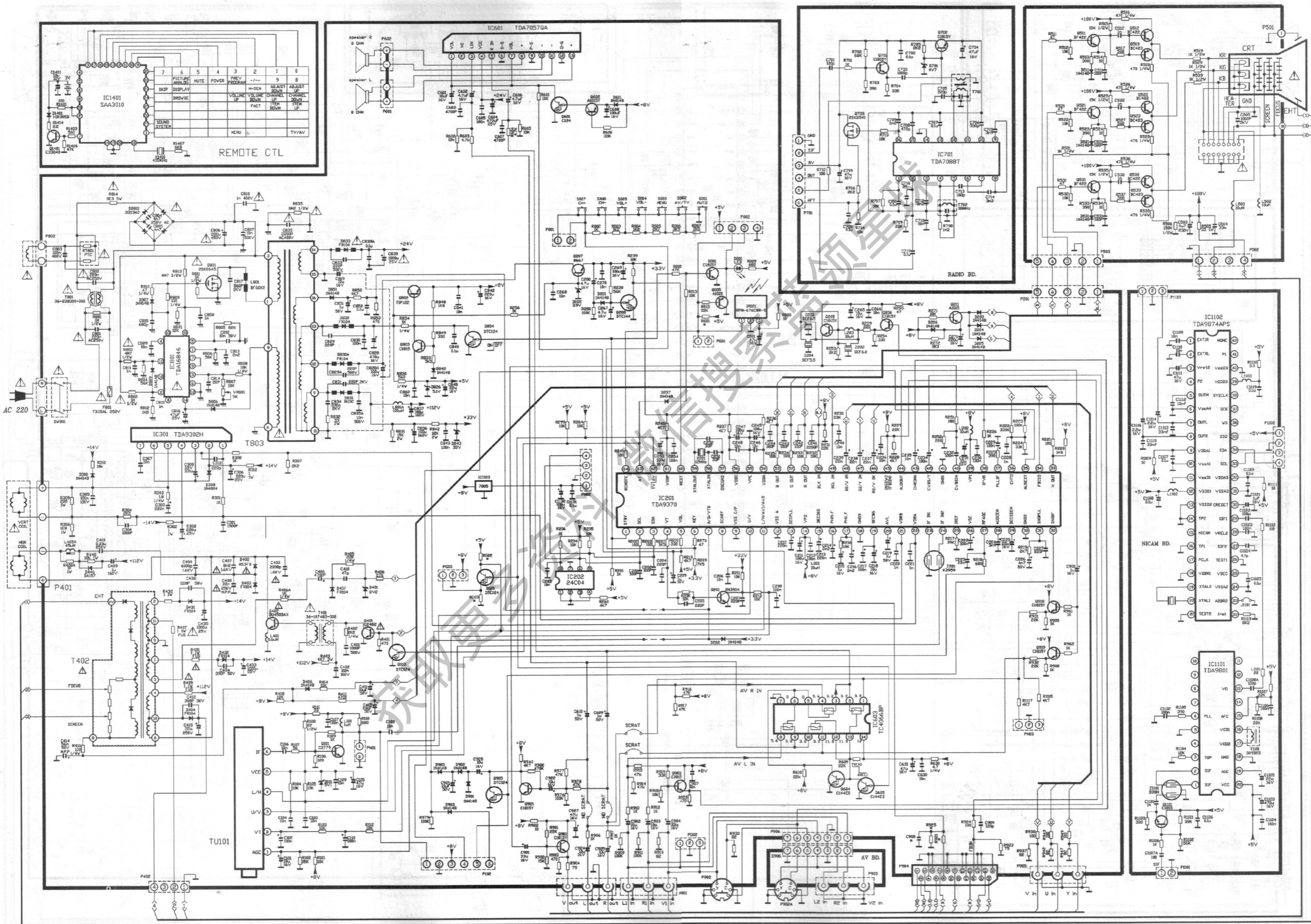
L-2165U4 型彩色电视机电路原理图
