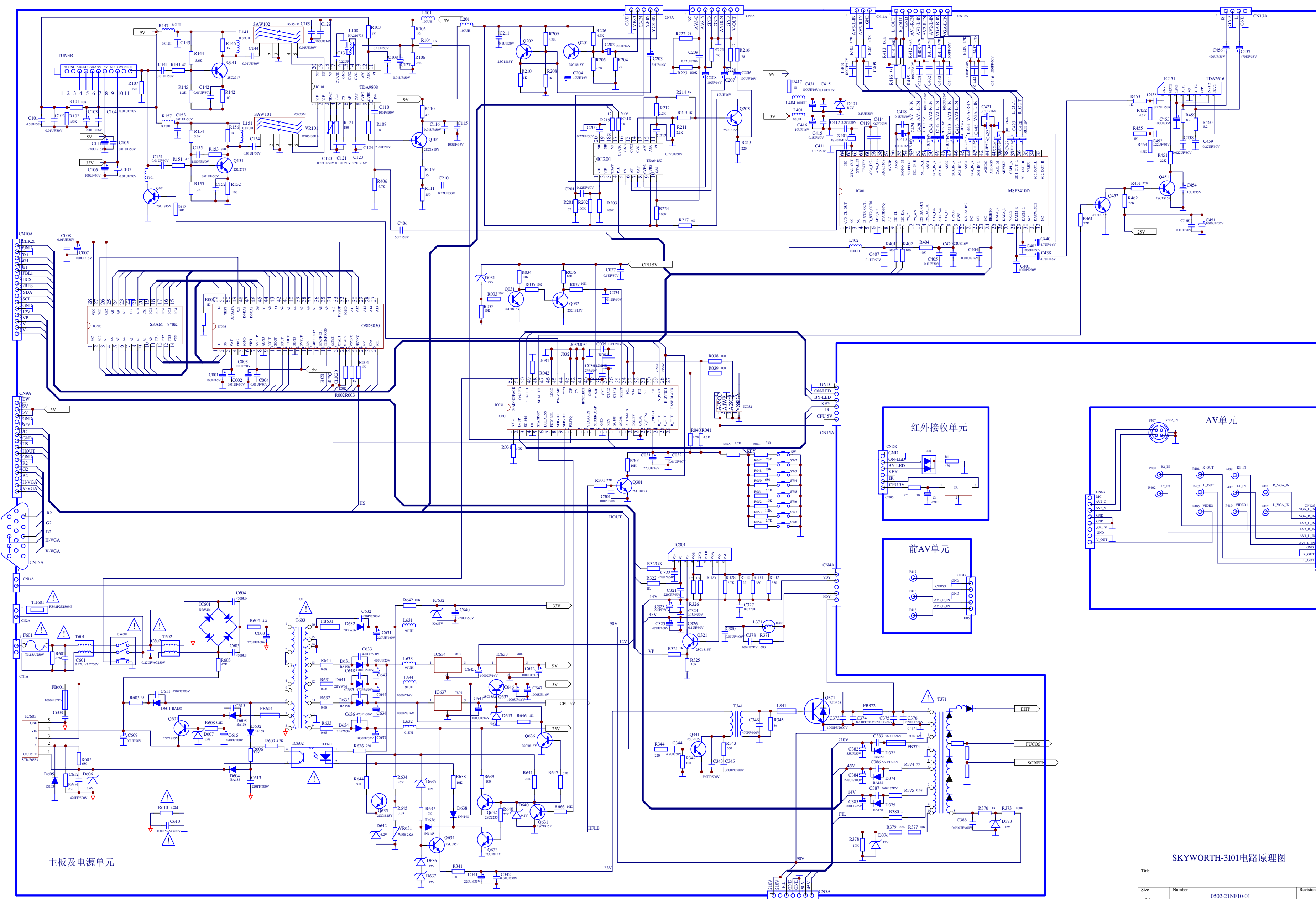
SKYWORTH-3101电路原理图 (主板单元、电源单元、AV单元及红外接收单元)
