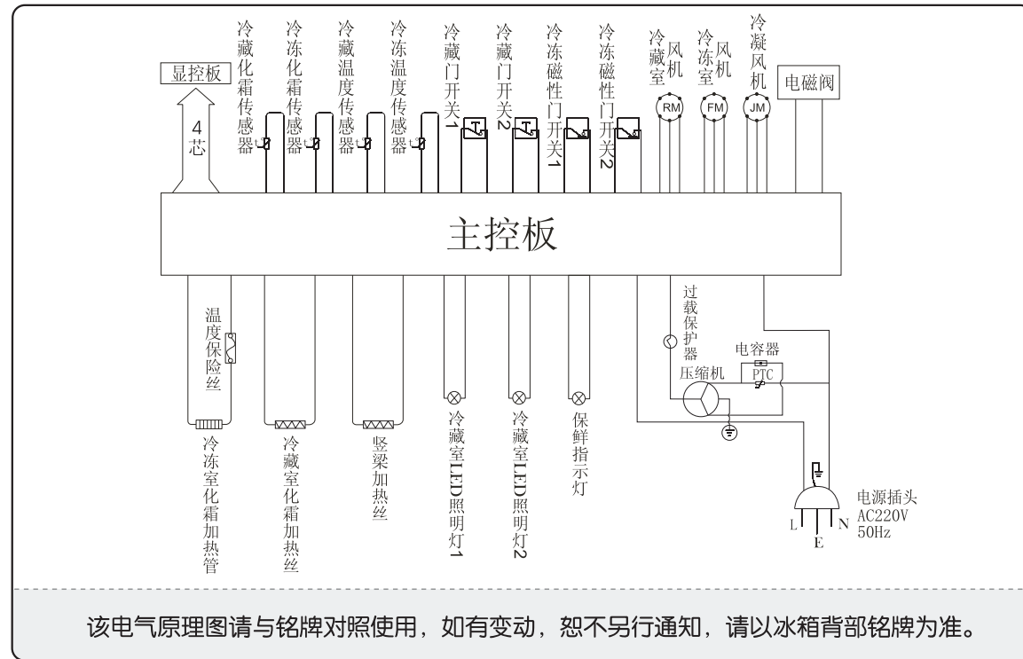
电路图 (BCD-401WMW/BCD-401WMGW)
