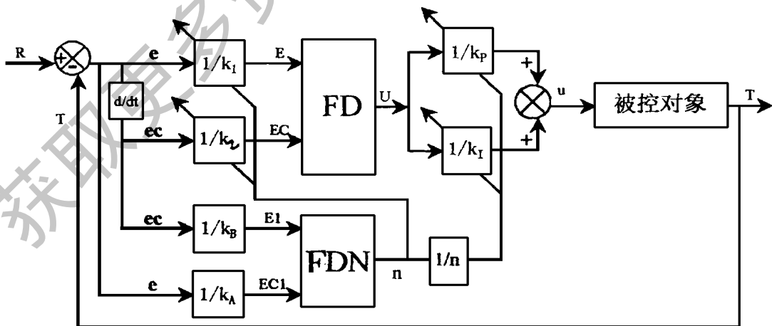
图 2 量子因子自调整 Fuzzy-Pi 控制系统框图
