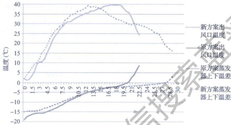
图9 出风口温度变化对比曲线
