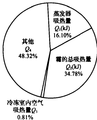
图8 新方案热量分配图
