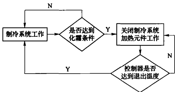
图1 化霜加热器常见断开控制逻辑
