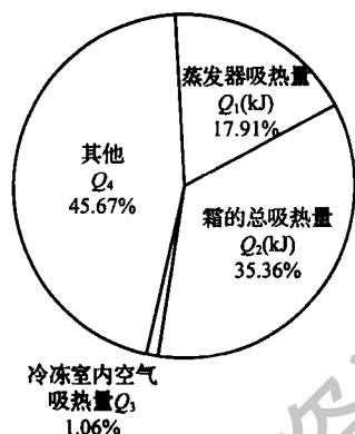
图 5 化霜热量分配示意图
