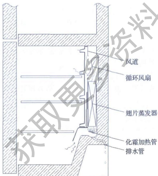
图2 风冷冰箱结构示意图
