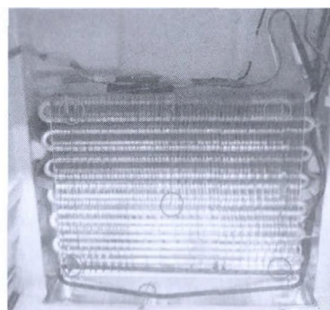
图3 蒸发器布点示意图
