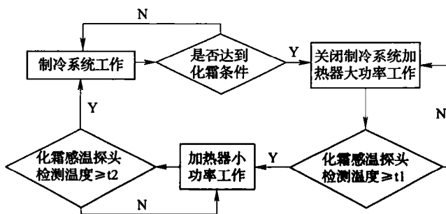
图 7 风冷冰箱化霜系统新工作方式
