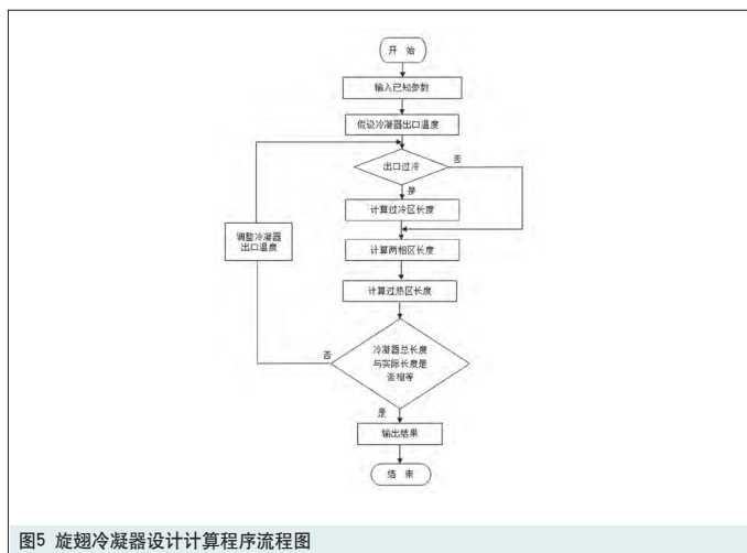
图5 旋翅冷凝器设计计算程序流程图
