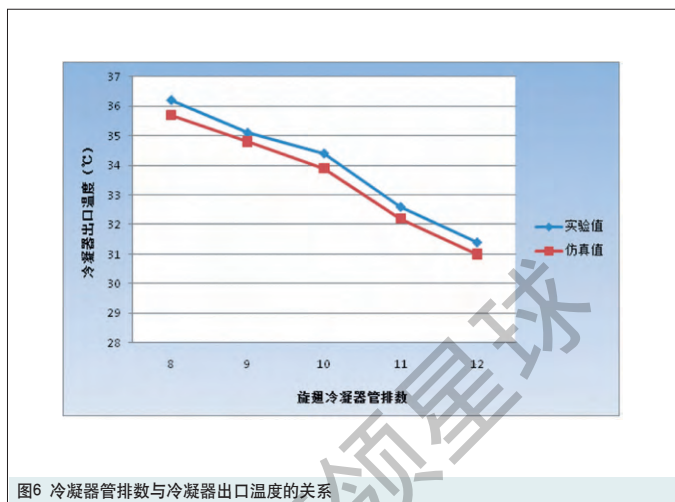
图6 冷凝器管排数与冷凝器出口温度的关系
