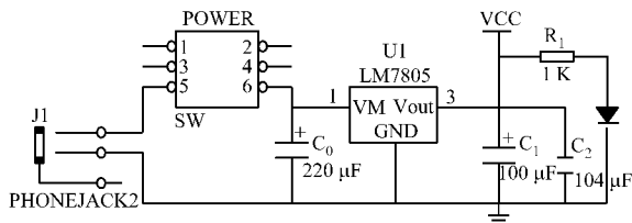
图 6 电源模块电路
