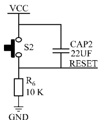
图 8 复位电路
