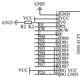
图 5 显示屏电路
