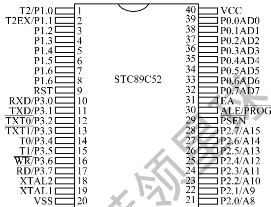
图 3 STC89C52 单片机引脚图
