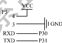
图 4 蓝牙接口图
