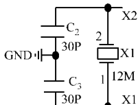
图 7 振荡电路
