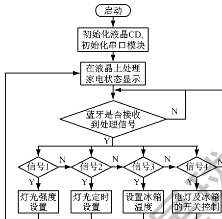
图 9 系统流程图
