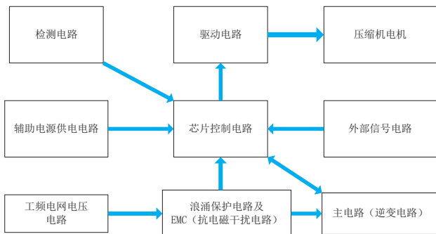
图 4 变频板硬件原理框图
