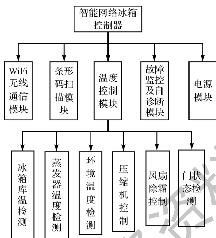
图1 系统模块图
