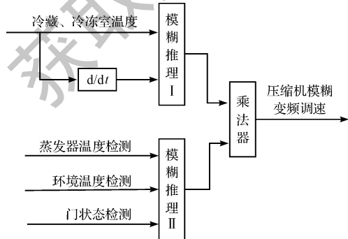
图 5 模糊控制器的结构框图
