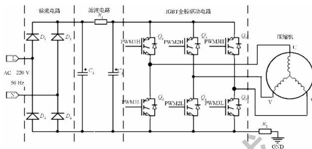
图2 变频调速电路原理图
