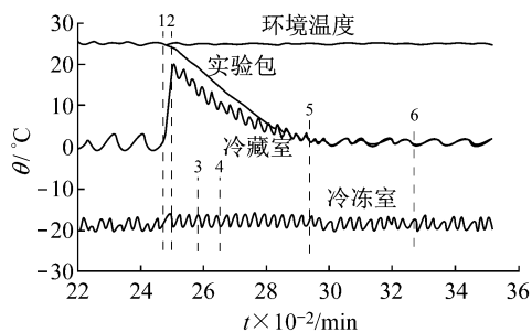
图3 实验3的温度曲线
