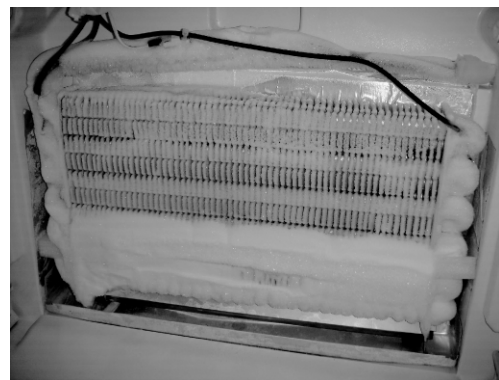
图9 改进前蒸发器结霜情况
