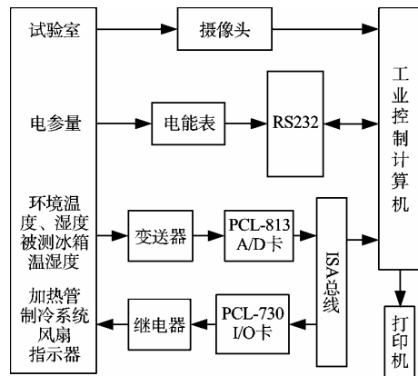
图 2 测试系统原理示意图
