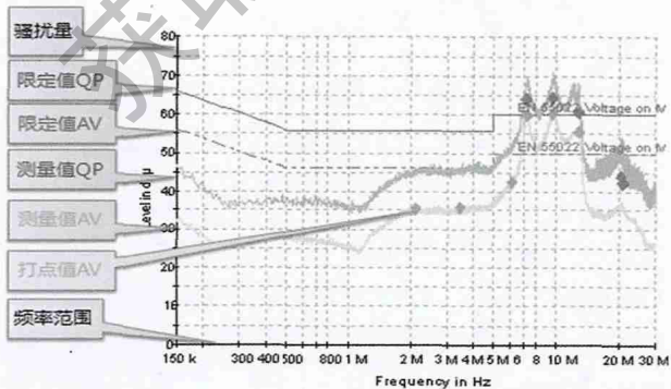
图 4 冰箱 EMI 实际测试干扰波形图
