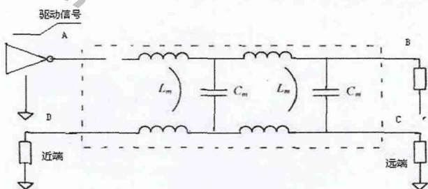
图3 耦合干扰示意图
