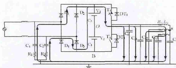
图 1 传导干扰示意图
