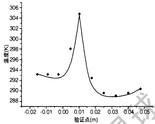
图 7 数值计算结果和实验数据的对比
