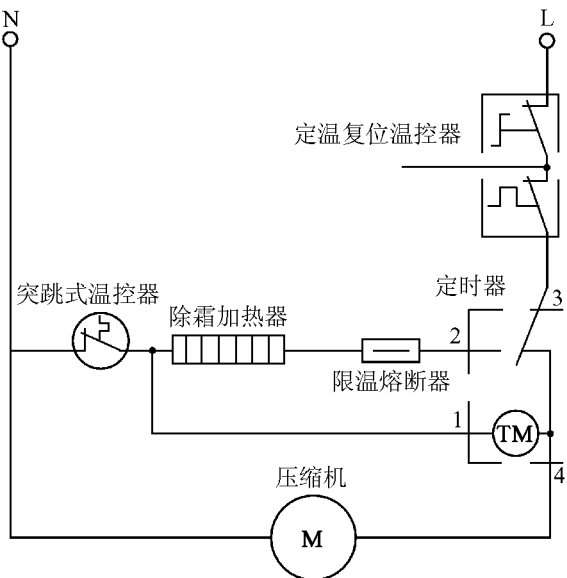
图 1 全自动除霜初步方案
