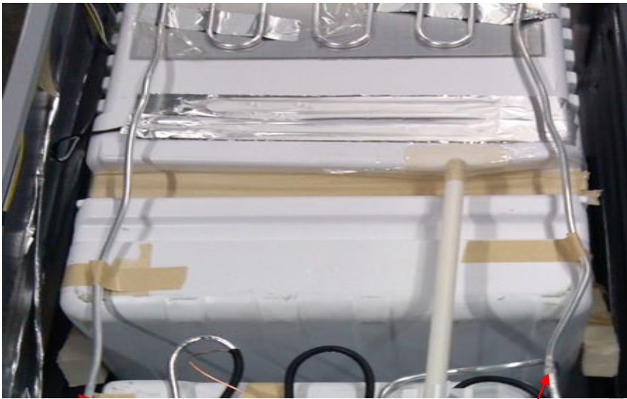
冷藏室蒸发器，铝铝焊接
