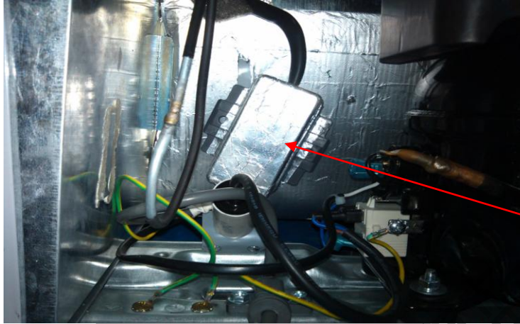
下图为接线盒线路，白色线为：控制压缩机线，蓝色线为：零线。棕色线为：火线。
