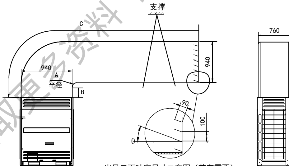
出风口百叶窗尺寸示意图 (若有需要)
