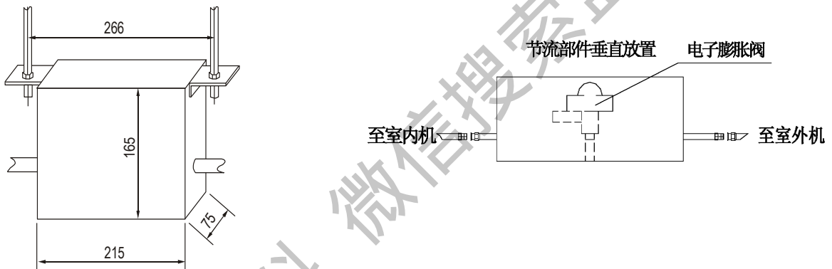
节流部件安装方式之一(仅供参考)
