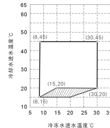
WPS.CDFST启动范围
