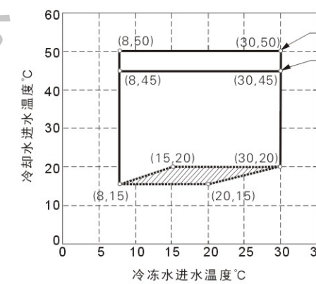
WPS.CFFST启动范围
