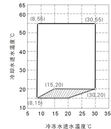
WPS.CDFHT启动范围
