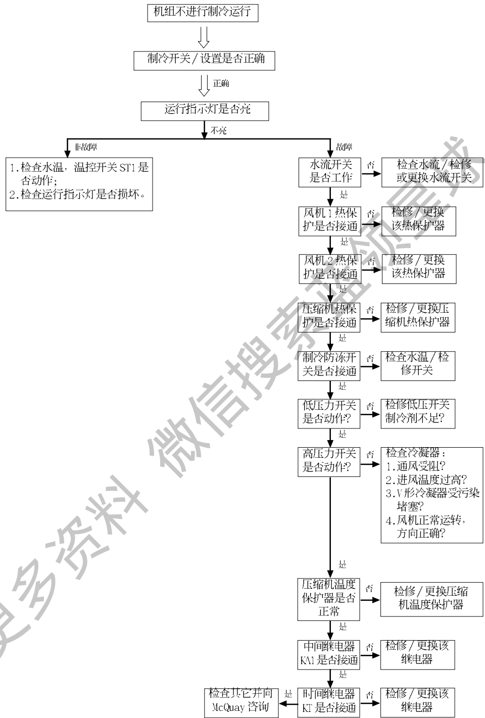
图 8-2 机组制冷运行故障分析流程图
