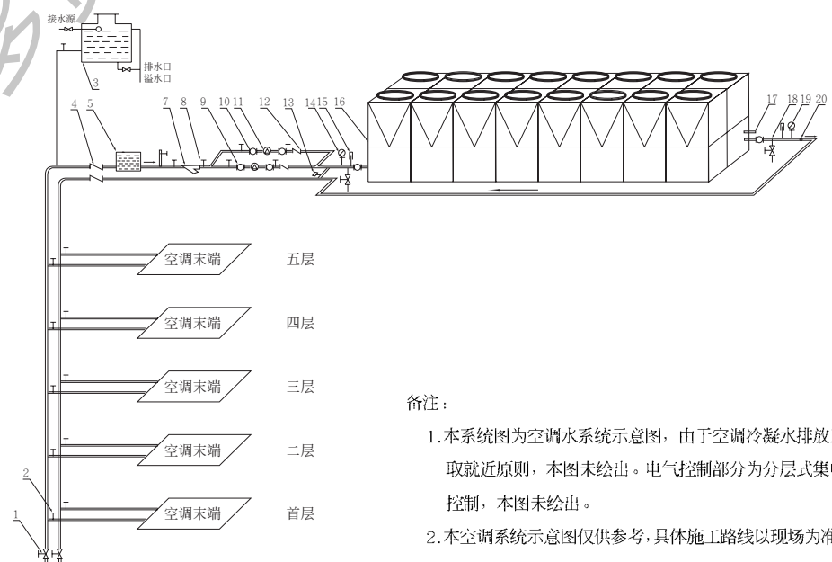
图 9-2 空调水系统图
