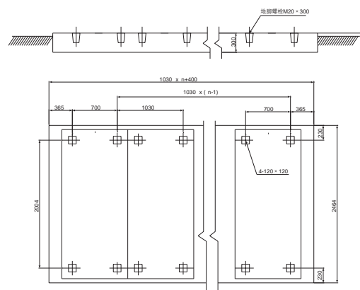
图 9-1：MAC 机组安装基础图
