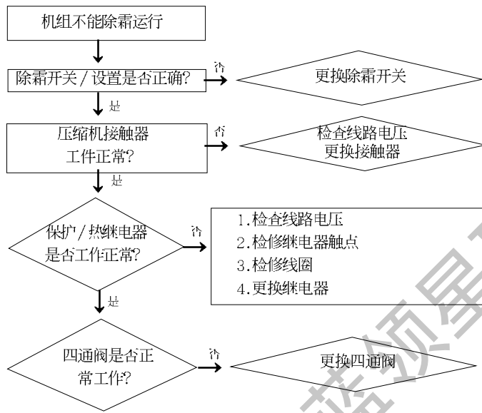
图 8-4 机组除霜故障流程图
