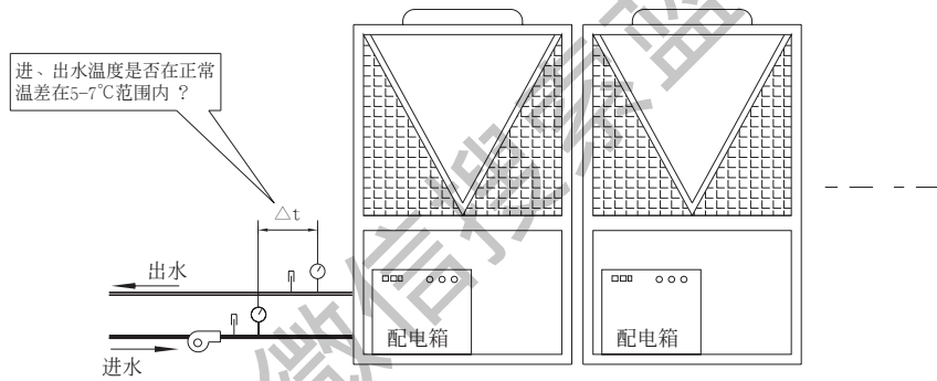
图7-5 进/出水温差检查
