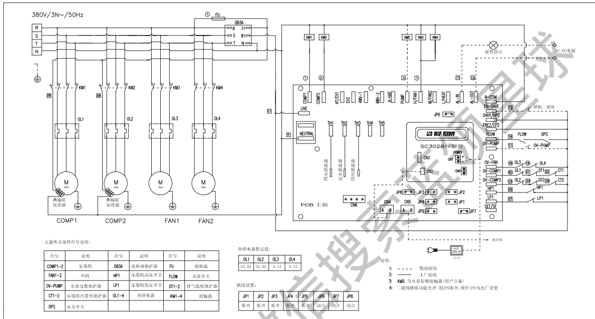
■ MAC260B (主机) 电路图
