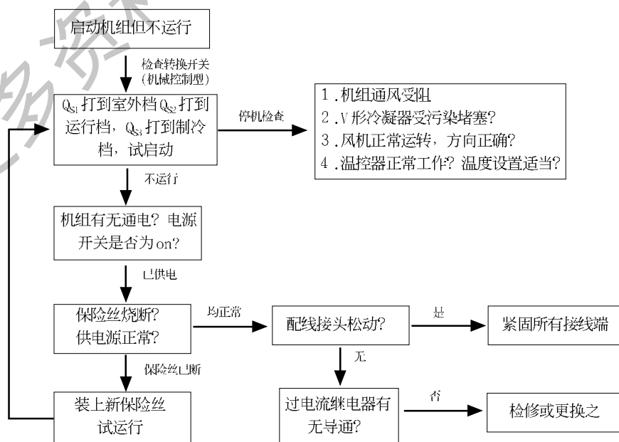
图 8-1 机组运行故障流程图
