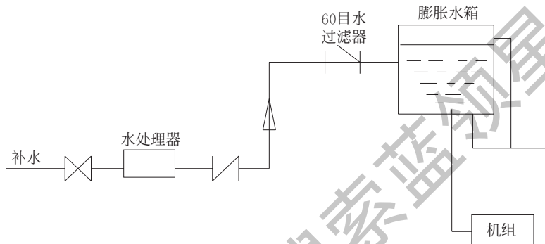
图 7-4 机组补水示意图
