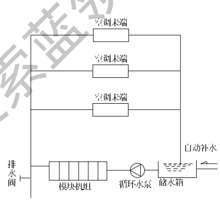
图4-2 开式水系统
