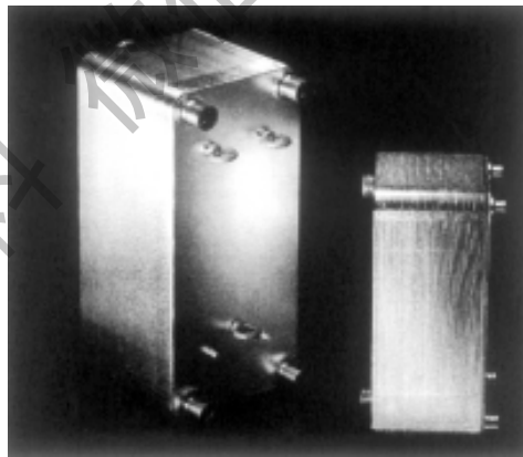
图 7-2 板式换热器外形
