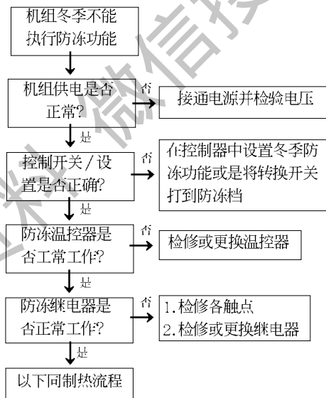
图 8-5 机组防冻故障流程图
