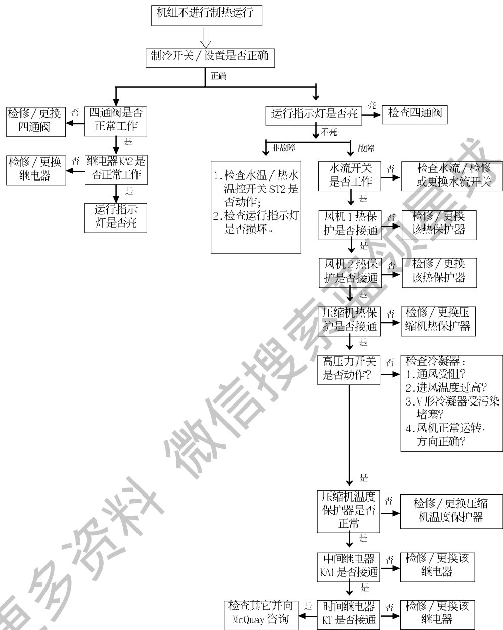
图 8-3 机组制热故障分析流程图
