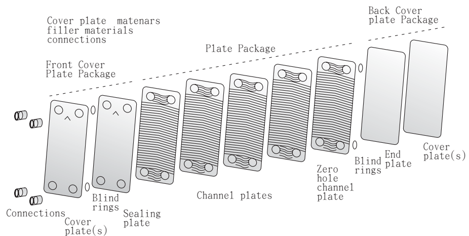
图 7-3 板式换热器结构分解图
