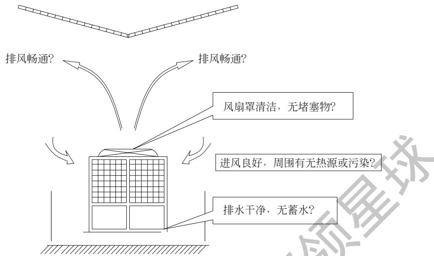
图 7-1 冷凝器检查与清洁
