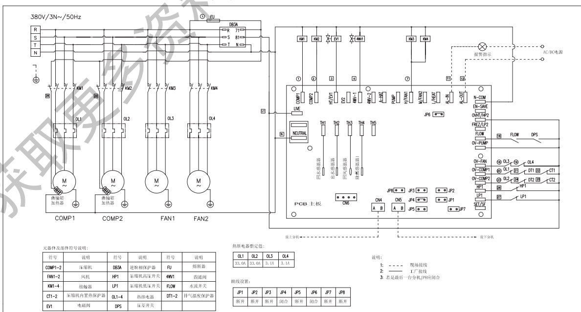
■ MAC260B (分机) 电路图
