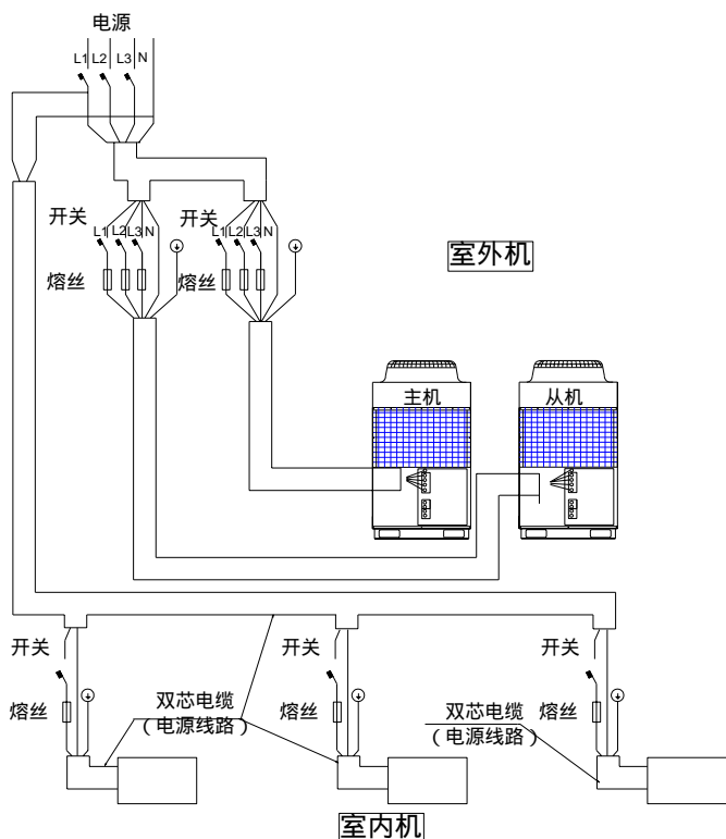
并联机组单独连接示意图<一>(适用于MDS260 ~ 320B(R))
