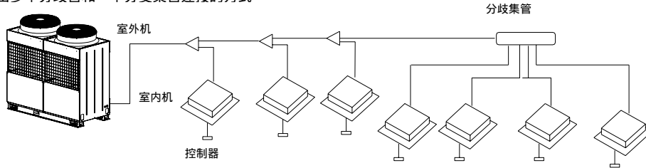
(3) 由多个分歧管和一个分支集管连接的方式
