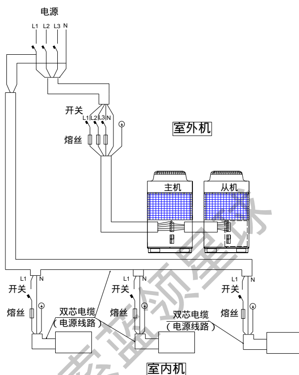
并联机组串联连接示意图<二>(适用MDS260 ~ 300B(R))
