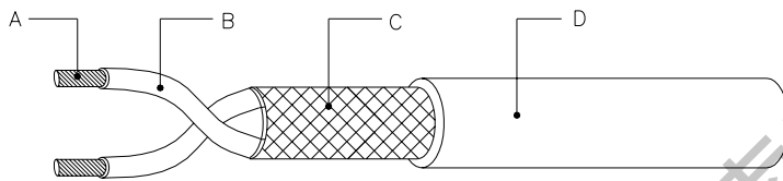
屏蔽双绞线图例
