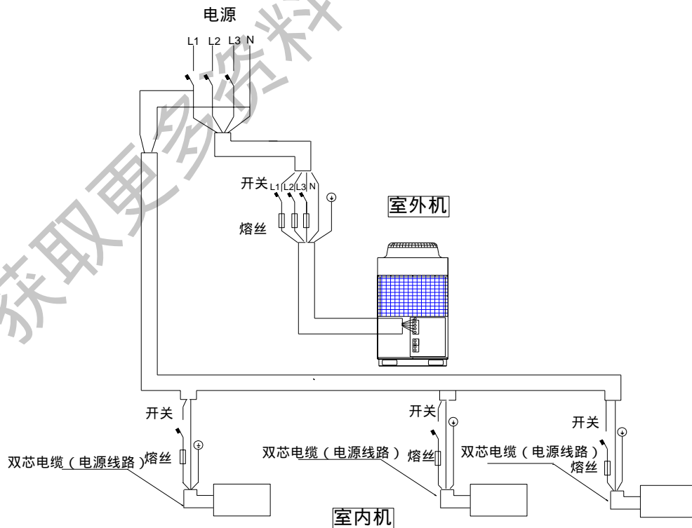
单机电气布线示意图(适用机型MDS080~240B(R))
