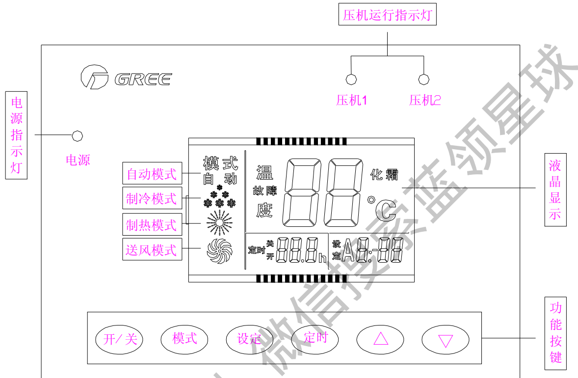
图 2.1.4 显示板 Z3010 外观及功能
