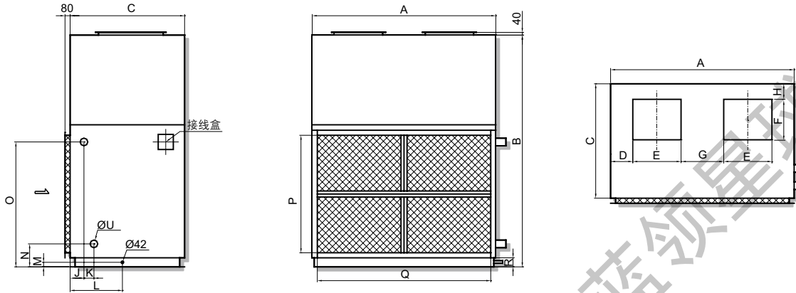
立式顶出风
