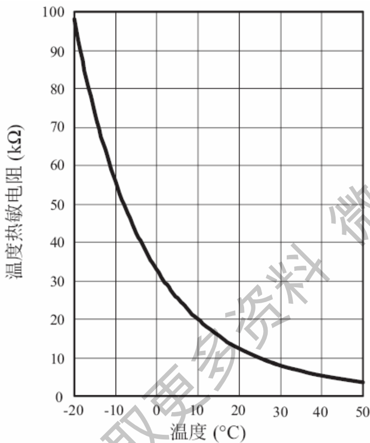
室外机环境温度 Tho-A
