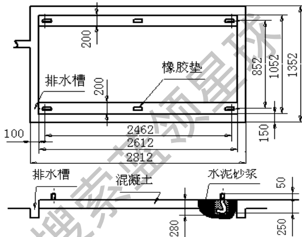
55、60、65kW 模块安装参考
