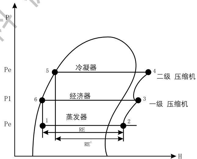
图3. 压-焓图
