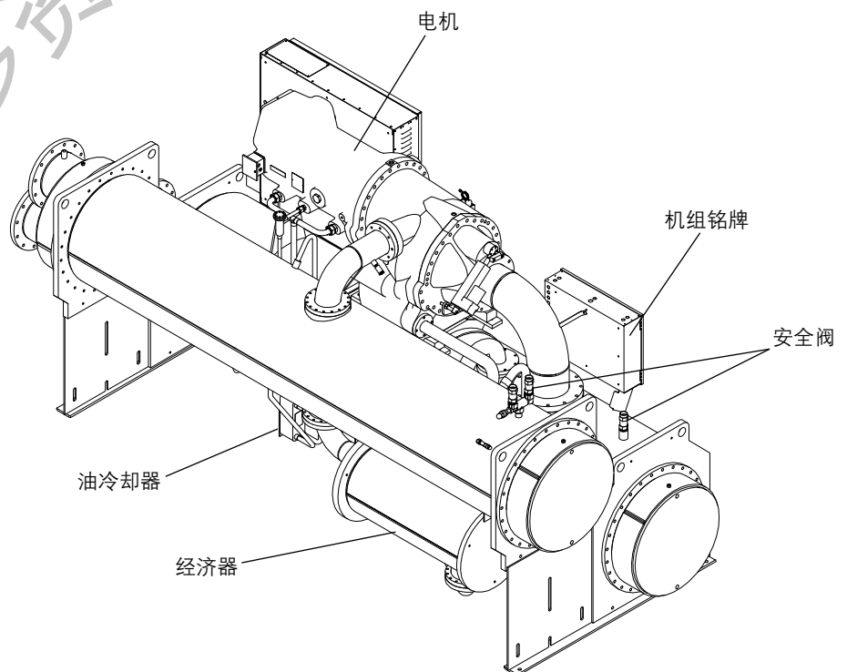
图2. 典型的CVGF机组部件分布 (后视图)
