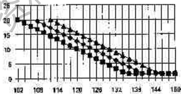
图22. 过载时间-跳闸与RLA百分比曲线
