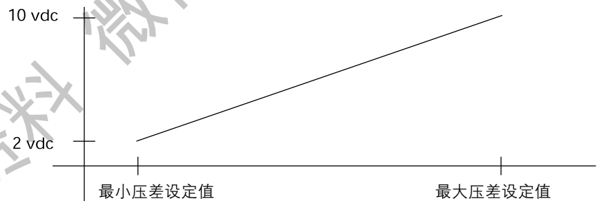
图19. 压差设置
