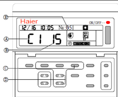
A A区数值 C 显示选择按钮 B B区数值 D 翻页按钮 E 模块地址号显示
