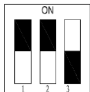
4#模块地址拨码
