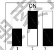
3#模块地址拨码
