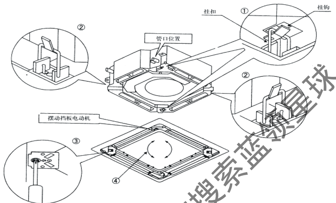
图 15：天花机面板安装顺序示意图
