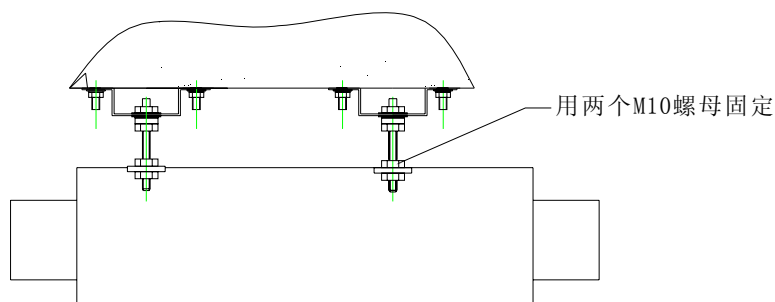
图 24: 低静压风管机吊装替代方式示意图
