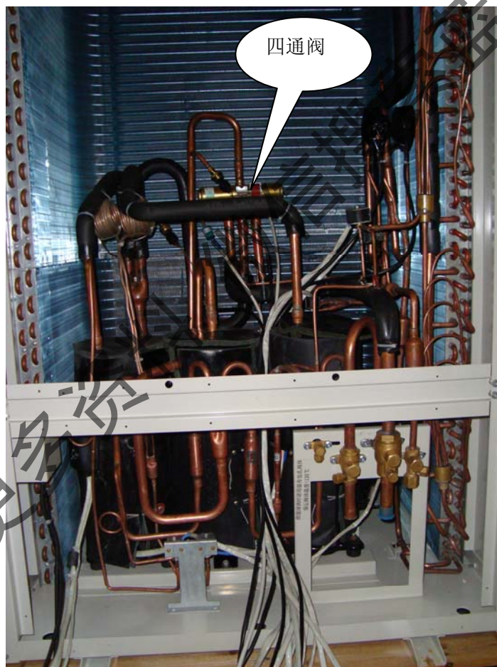
图 9: CMV-[V]直流变频模块式多联机四通阀位置示意图
