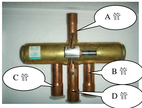
图7: 四通阀的示意图
