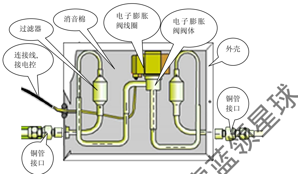
图 17 电子膨胀阀部件内部结构示意图
