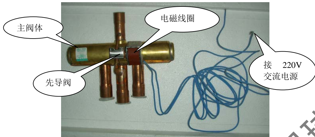
图 4：四通阀实物图
