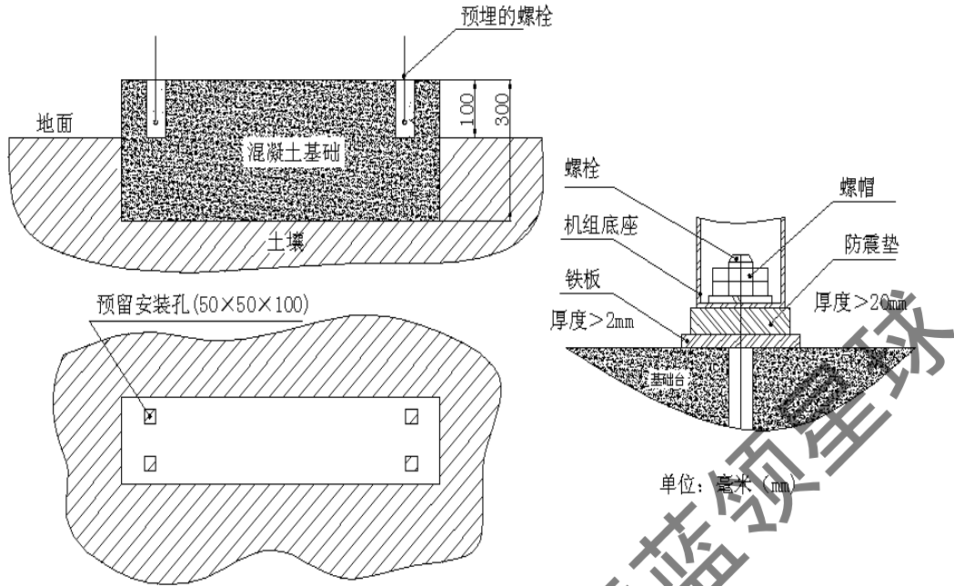
图 4：室外机混凝土安装基础示意图
