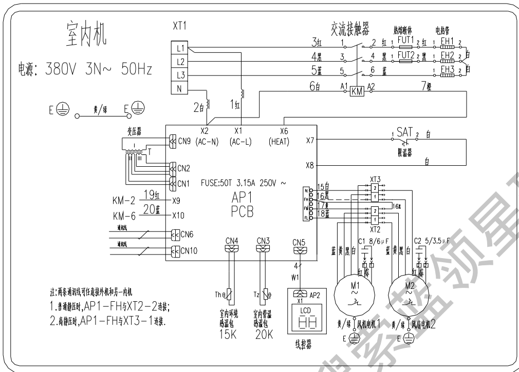
GMV-J25P/D、GMV-J35P/D 电路图
