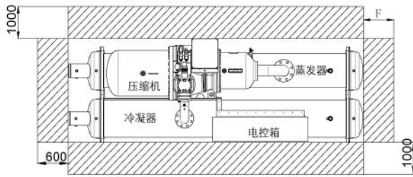
单系统机组预留维修空间
