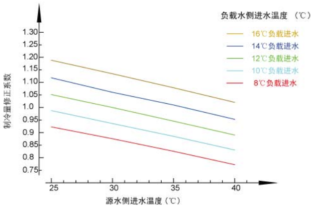
说明:此图以水环式工况标准制冷时制冷能力系数为1
