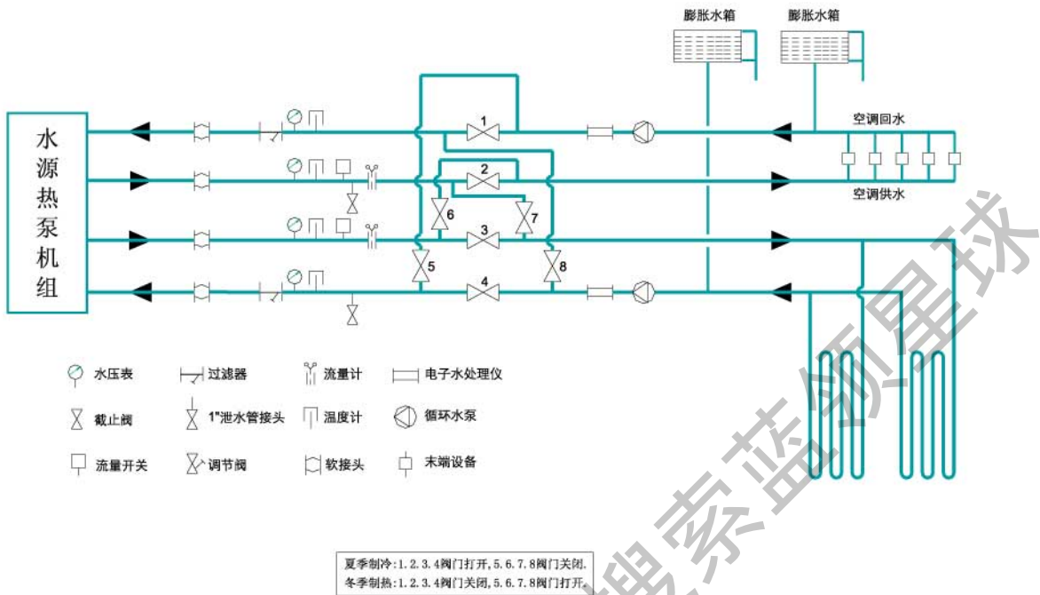
附图3: 机组使用地下环路工况原理图--方案3(水系统部件由现场安装,不随机供货)
