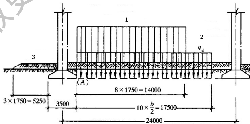
图 15 地面荷载计算示意
