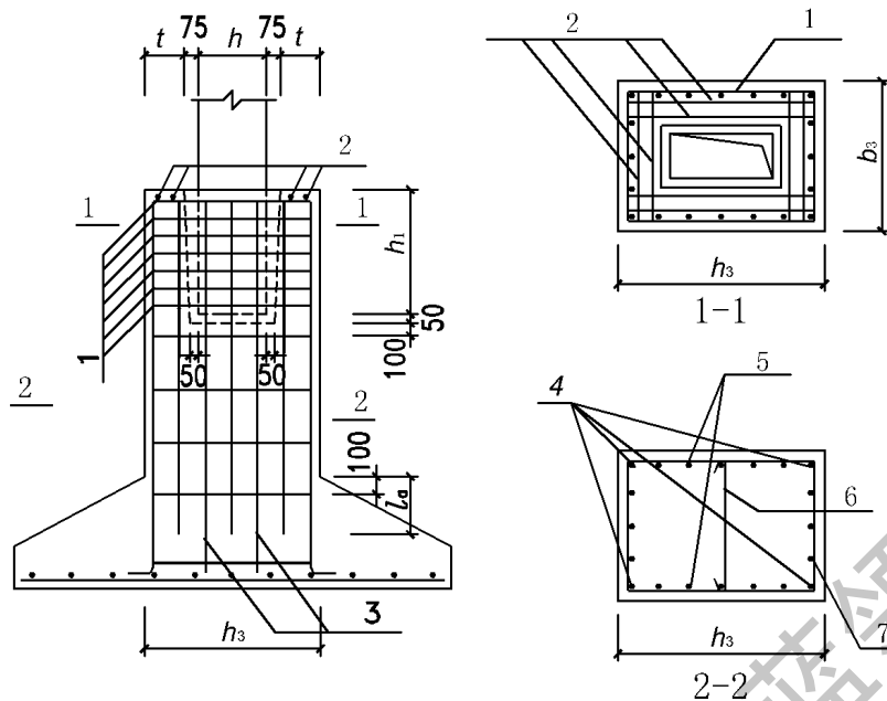
图 8.2.5-2 高杯口基础构造配筋
