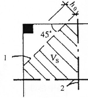
图 23 角柱(筒)下筏板验算剪切部位示意 1-验算剪切部位; 2-板格中线
