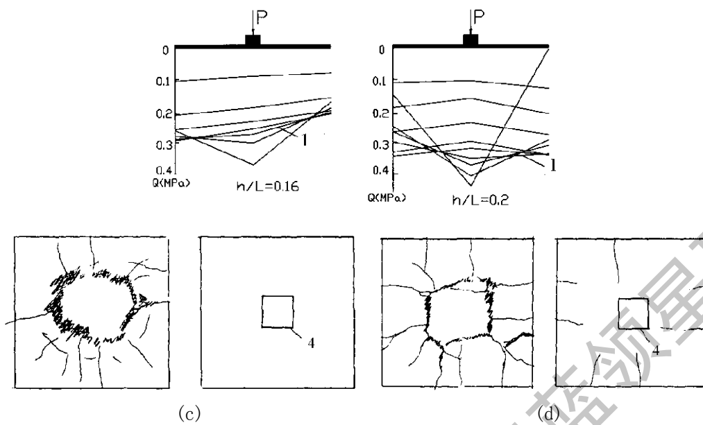
图 18 不同宽高比的基础板下反力分布
