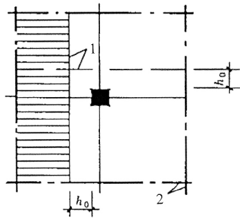
图 22 内柱(筒)下筏板验算剪切部位示意 1-验算剪切部位; 2-板格中线
