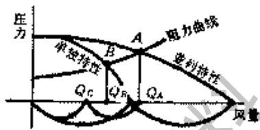
图 2.3.4-3 风机并联运行特性
