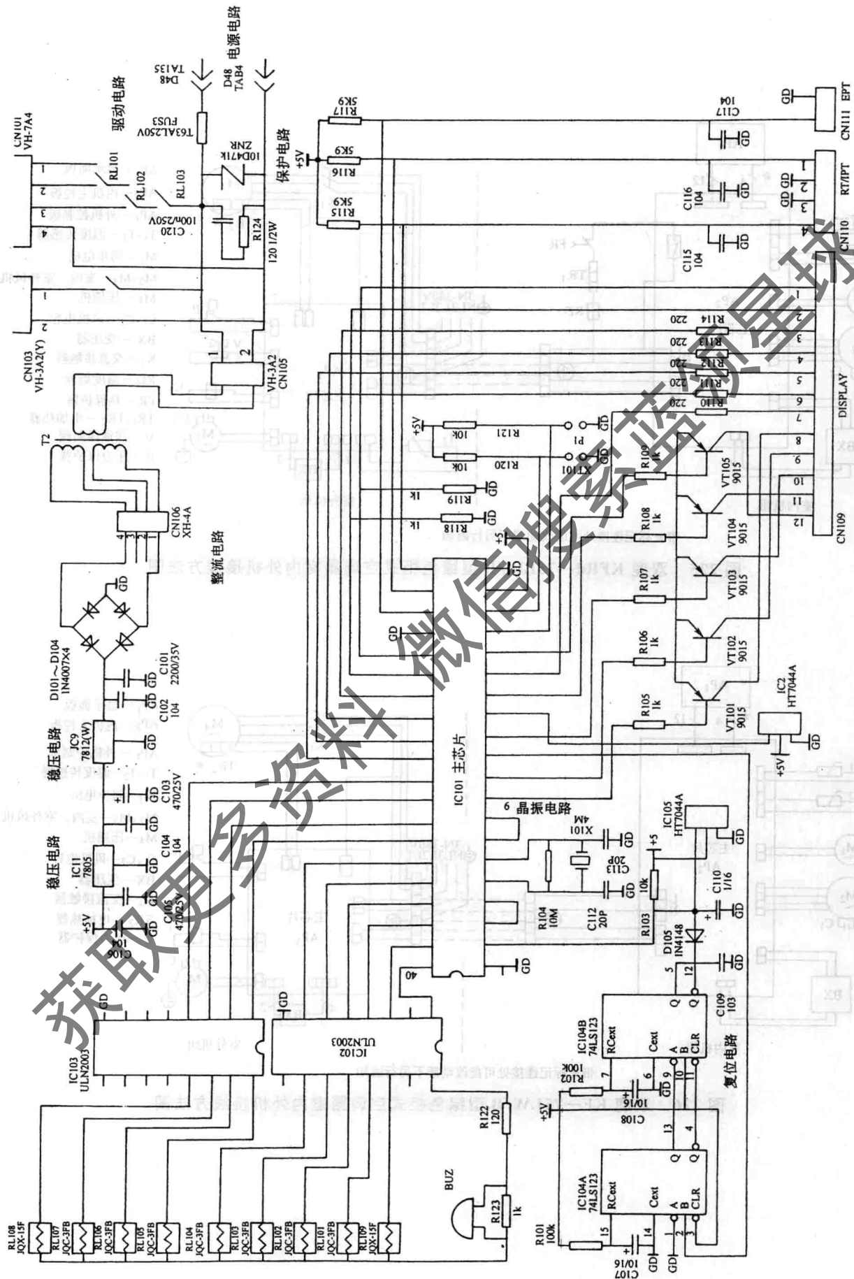
图 224 双鹿 KFR—48LW/A、KFRd—75LW/A 型柜式空调器室内机微电脑控制电路图
