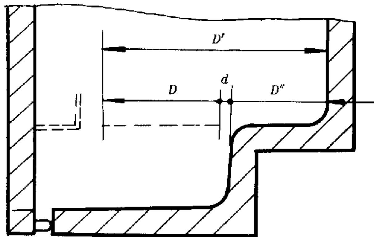
图 B4 搁架面积确定的示例
