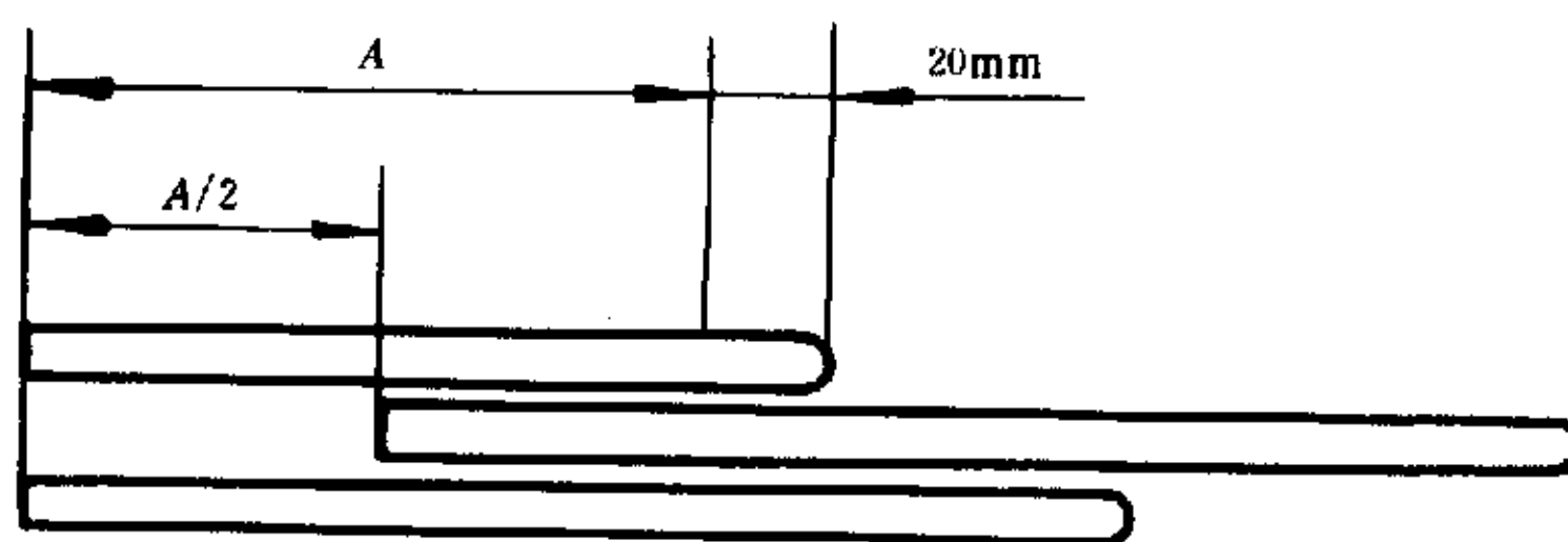
图8 无限位器时活动部件的试验位置
