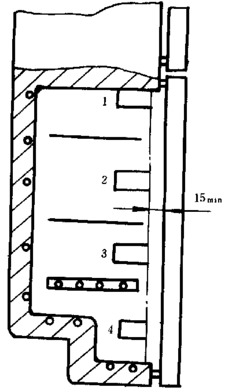
侧剖视图
