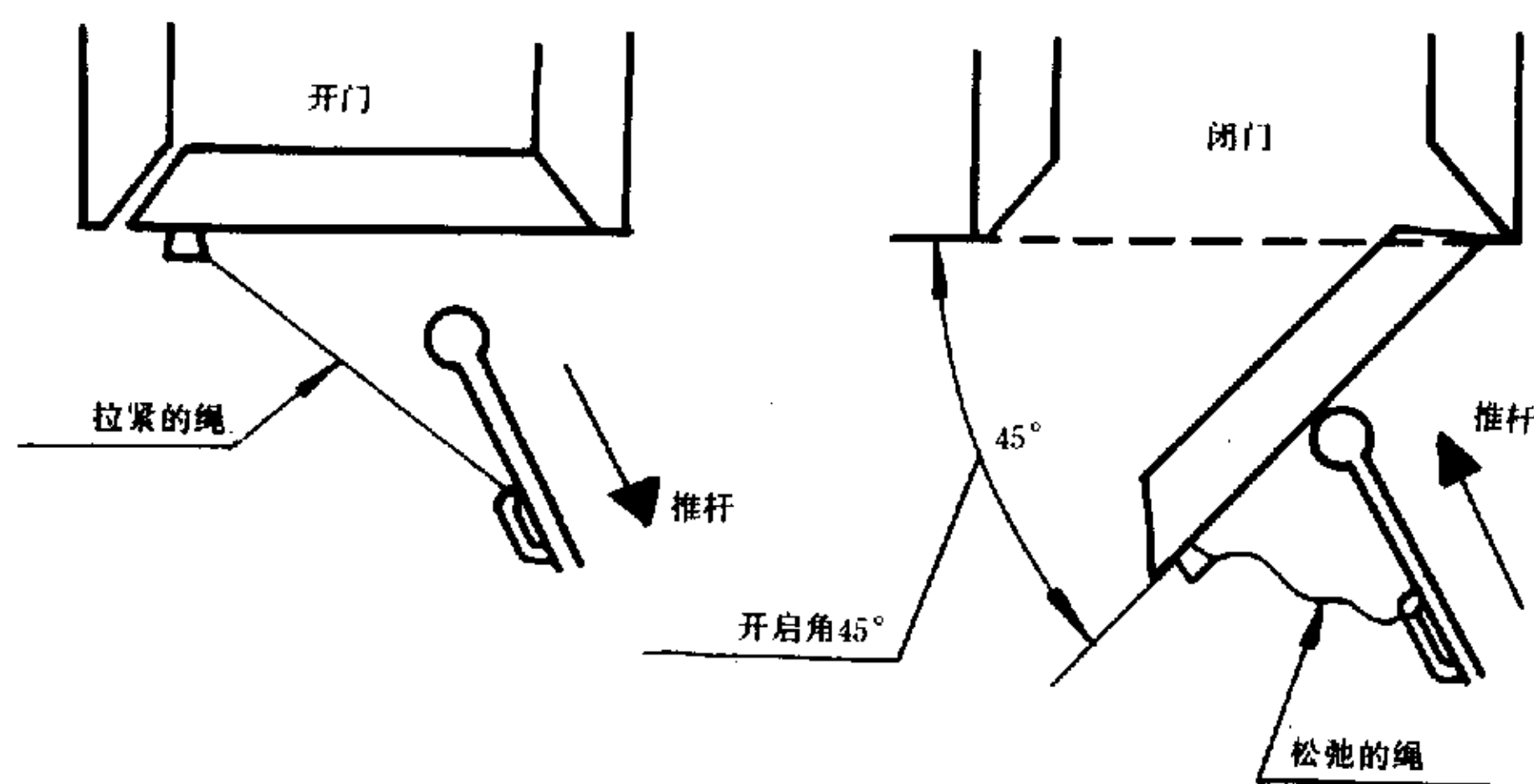
图7 外门开闭示例
