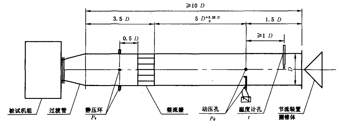
图 A.1 多个喷嘴空气流量测量装置
