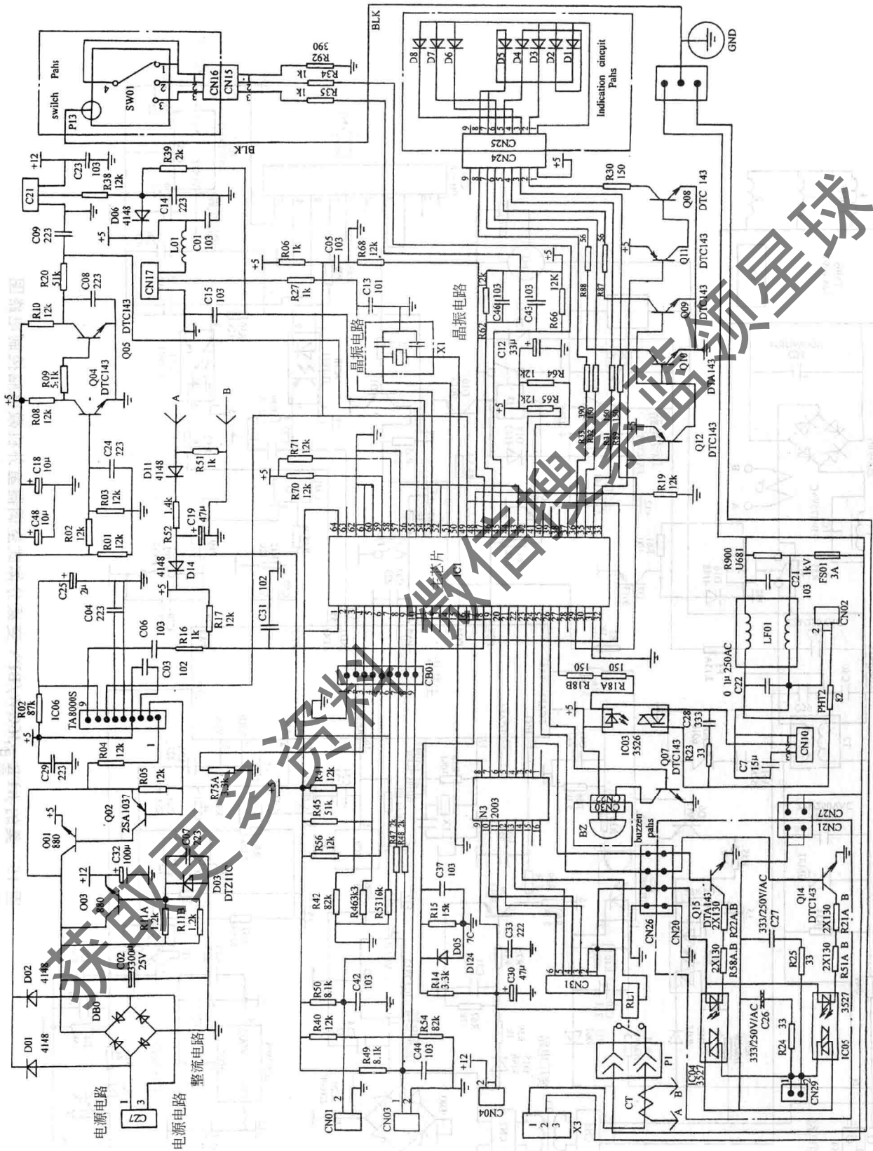
图 16 美的 KFR-43GW/Y 分体式空调器微电脑控制电路图
