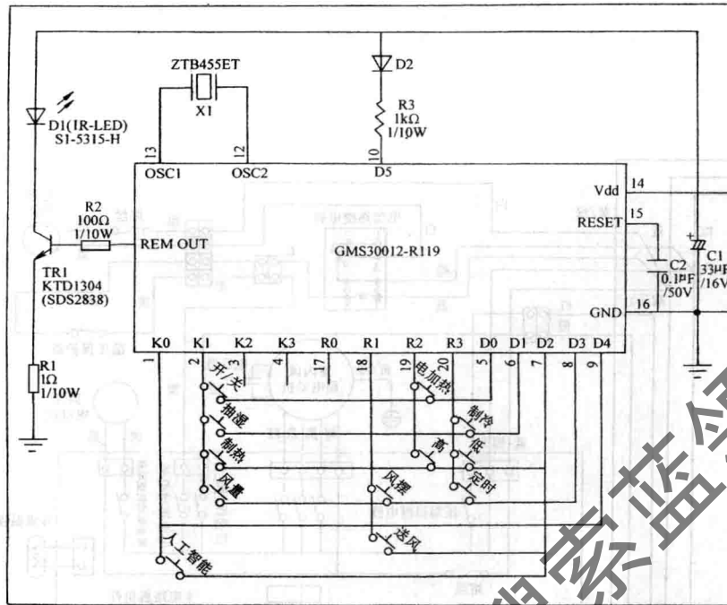
图 26 松下 CU—C180FW、CS—A180KW—1、CS—A270FW 空调器遥控器控制电路图
